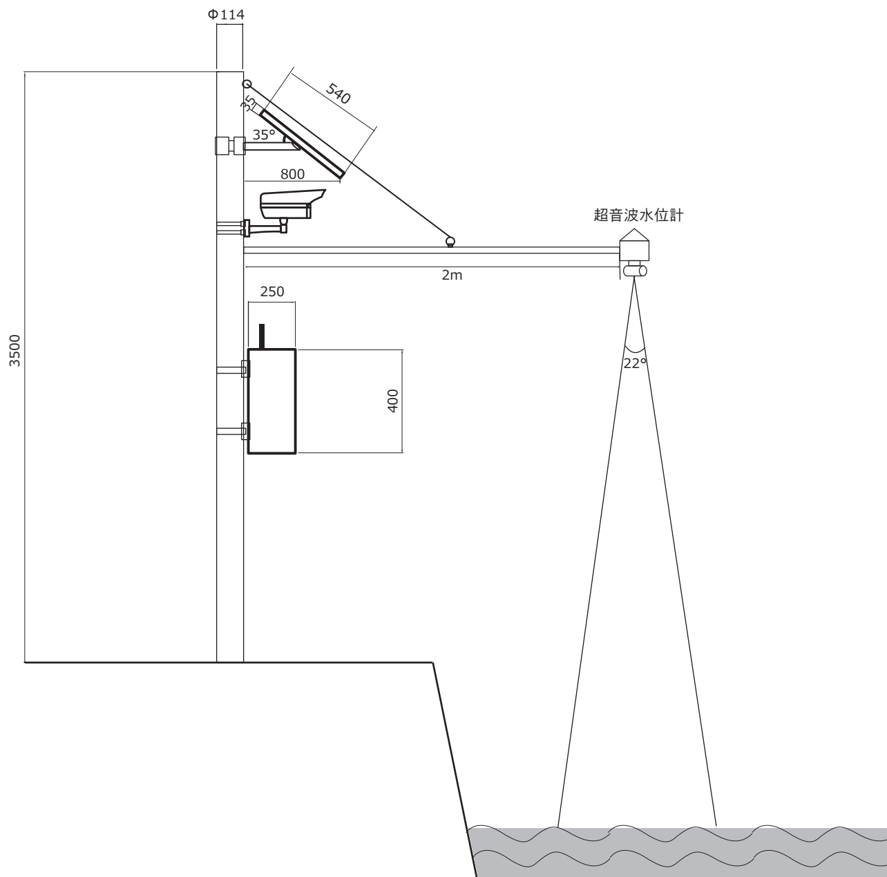
概観図
